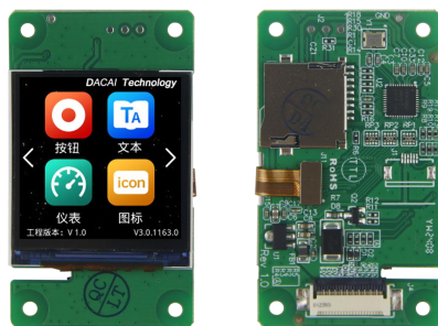
图 1-2 1.5 寸无触摸参考图
