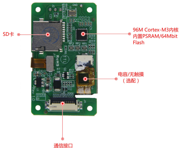
图 1-3 硬件配置图
